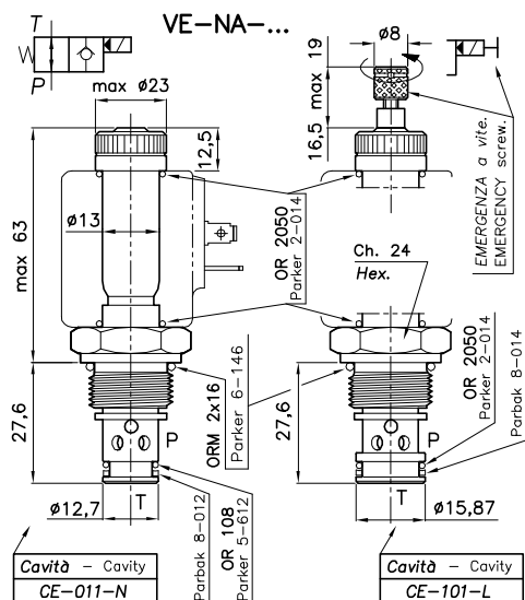
CAVITA' CAVITY CE.011-N
