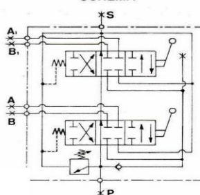
SCHEMA
